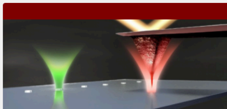
MICROSCOPIA A FORZA ATOMICA IN AMBIENTE LIQUIDO (OPT-ACT) Azionamento ottico di cantilever
